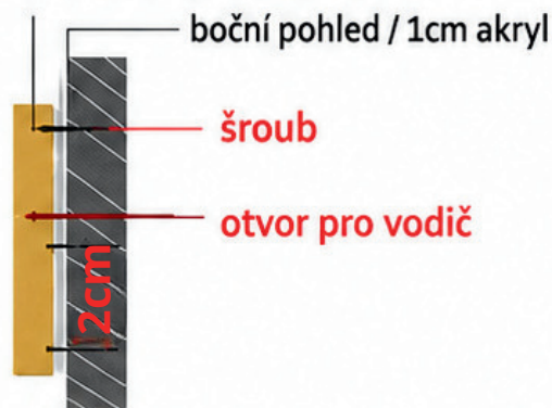
boční pohled instalace
